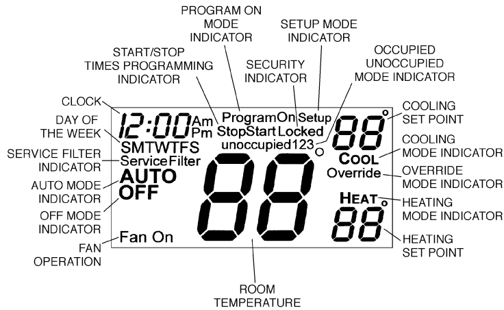
Fig. 1 — Thermostat Display
